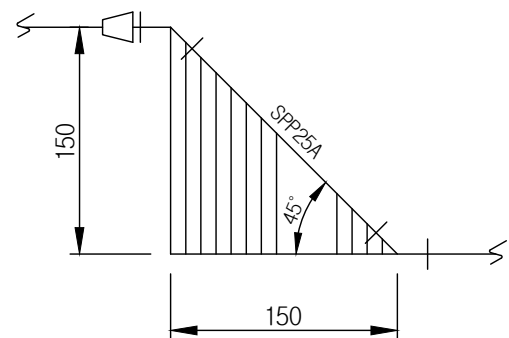
B - B' 단면도
